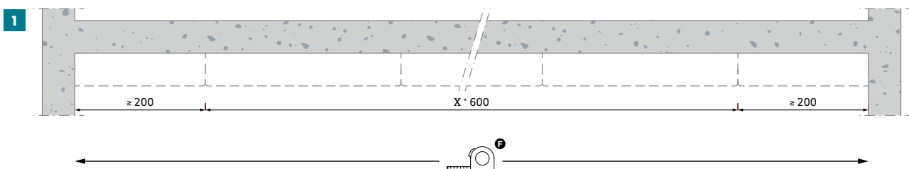
Doorsnede A A
